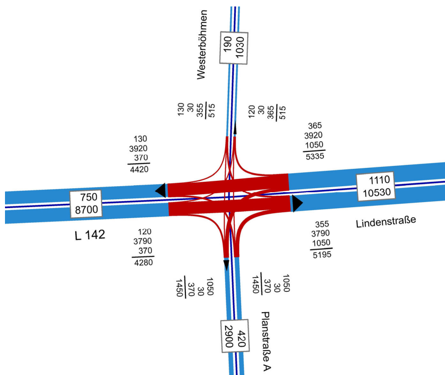
Bild 10: Verkehrsströme im Planfall 2 am Knotenpunkt Lindenstraße (L 142) / Westerböhlen / Planstraße A [Kfz/24h]
