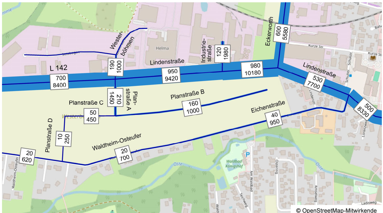
Bild 8: Prognosebelastungen 2035 im Planfall mit Bebauungsplangebiet Nr. 53 [Kfz/24h]
