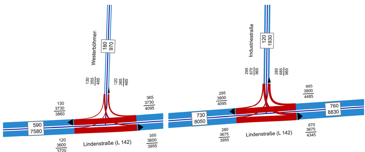
Bild 3: Verkehrsströme an den Knotenpunkten Westerböhlen (1) und Industriestraße (4) [Kfz/24h]
