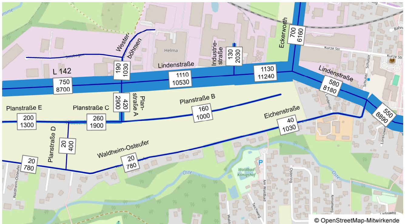
Bild 9: Prognosebelastungen 2035 im Planfall 2 mit B-Plangebiet und Erweiterungsfläche [Kfz/24h]
